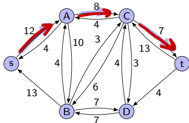
Restnetzwerk G_f |f| = 17
