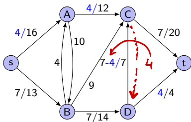
Flussnetzwerk G für |f| = 11
