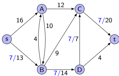
Flussnetzwerk G ( |f| = 7 )
