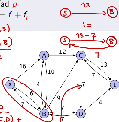
Restnetzwerk G_f für |f|=7
