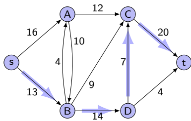
Restnetzwerk G_f (für |f| = 0 )
