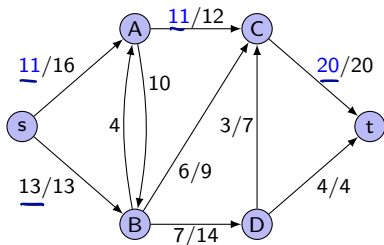
Flussnetzwerk G |f| = 24
