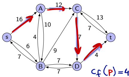
Restnetzwerk G_f
