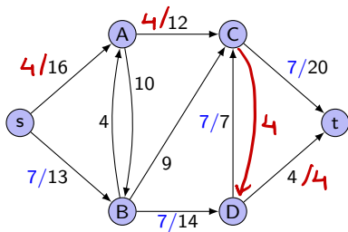
Flussnetzwerk G
