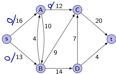
Flussnetzwerk G |f| = 0
