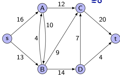
Restnetzwerk G_f für |f| = 0
