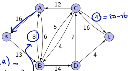
Restnetzwerk G_f
