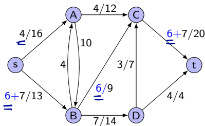
Flussnetzwerk G
