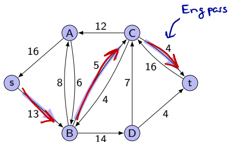
Restnetzwerk G_f
