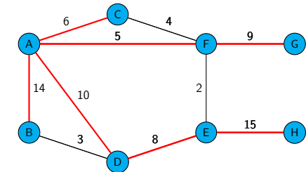
Breitensuchbaum (von A gestartet) Gesamtgewicht: 67
