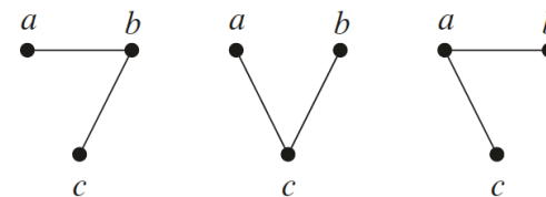
3 Spannbäume für n=3 Knoten
